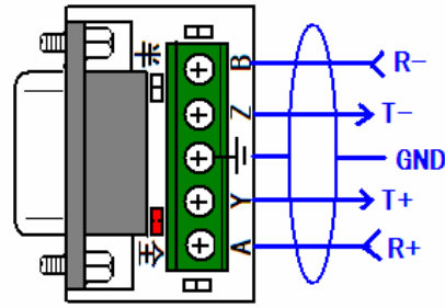
RS-422 全双工
