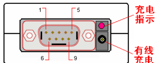
针 RS-485/422
